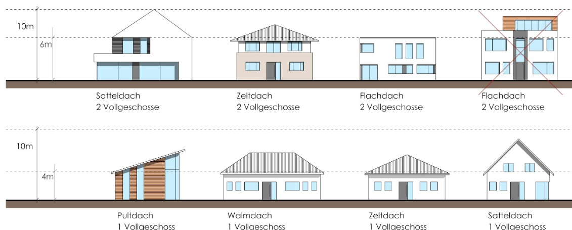
Denkbare Gebäudetypen
